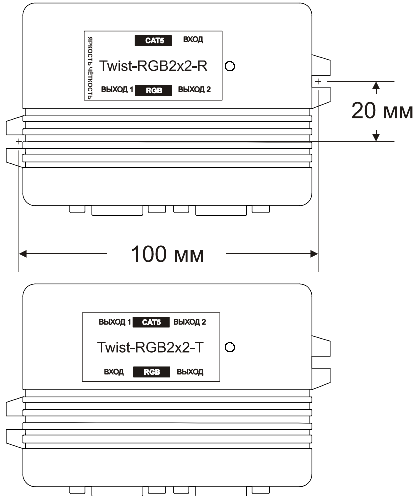
Рис 1. Общий вид кодера и декодера. Показаны установочные размеры для кодера и декодера
