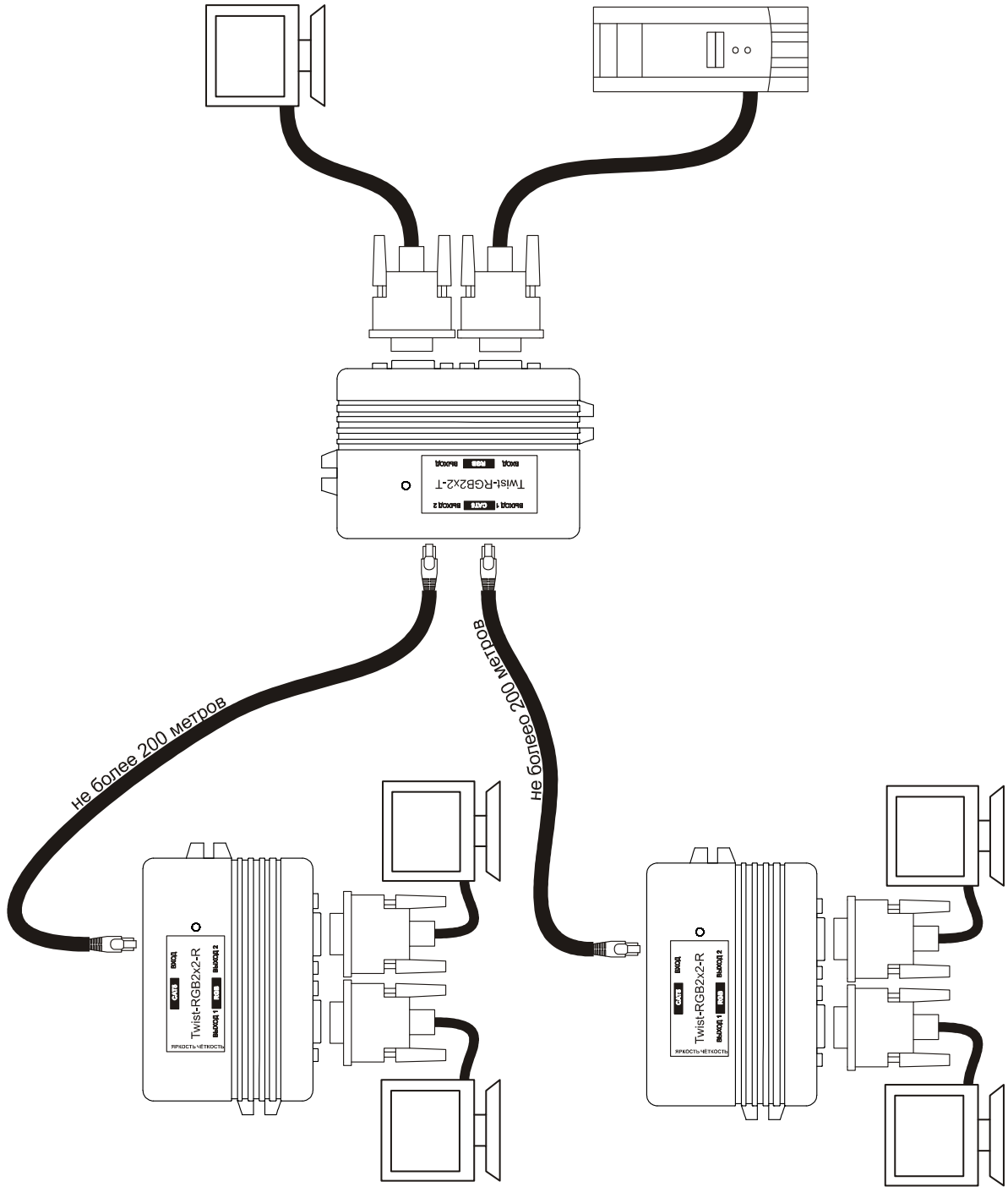
Рис 2. Схема подключения кодера и декодера
